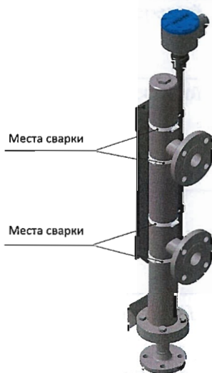
Рисунок 2 - Места фиксации уровнемера
