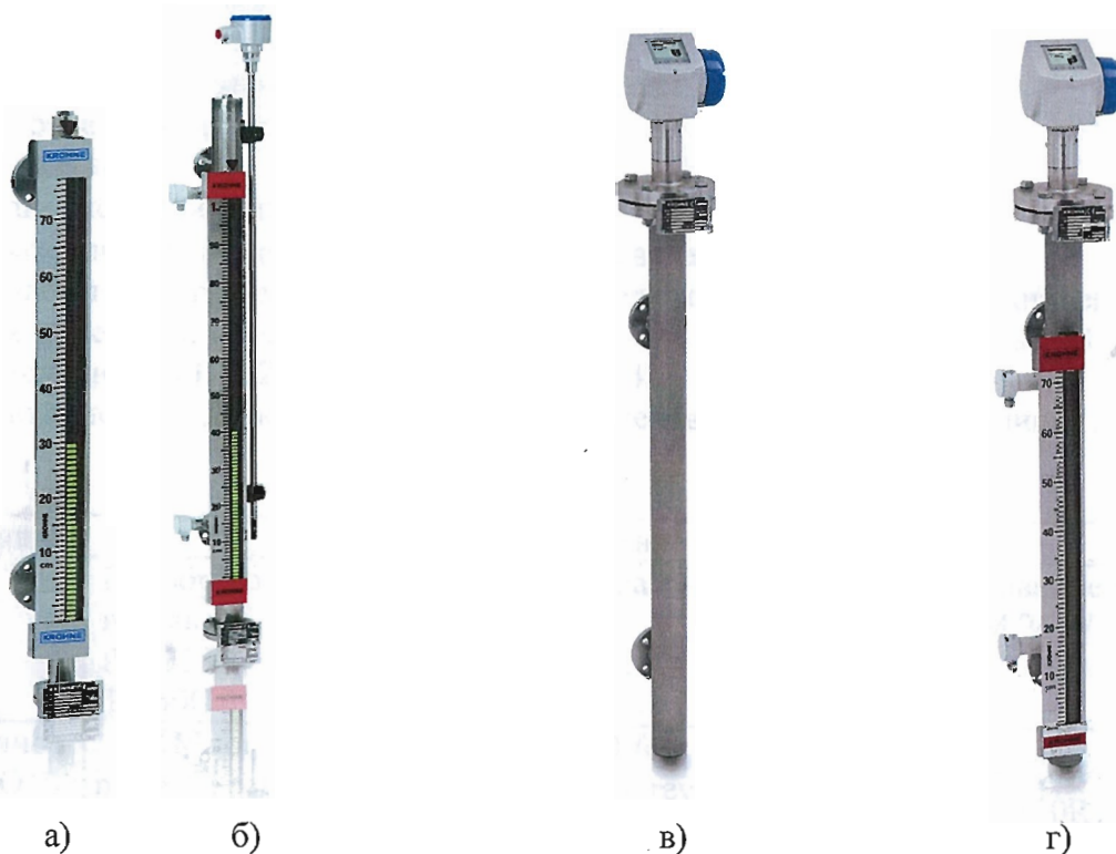
Рисунок 1 - Уровнемеры ВМ 26
