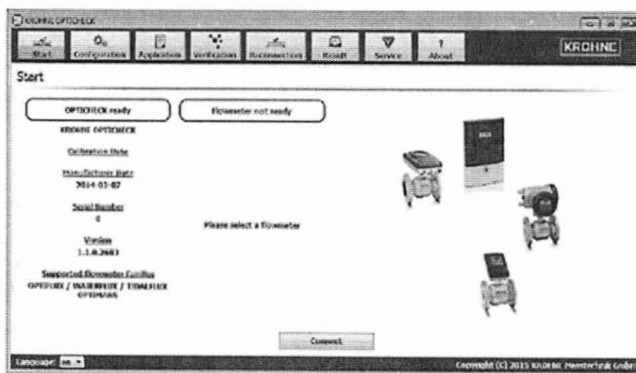
Рисунок 3 – Стартовое окно
