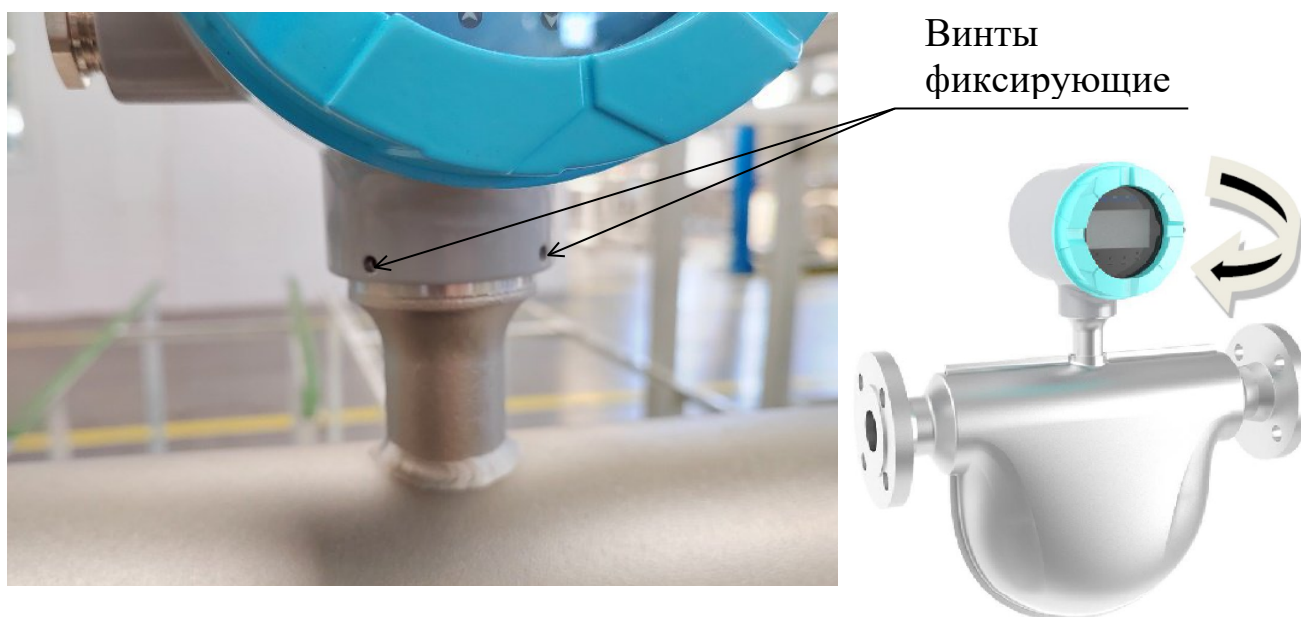
Рисунок 7 – Поворот корпуса преобразователя сигналов WMC-40
