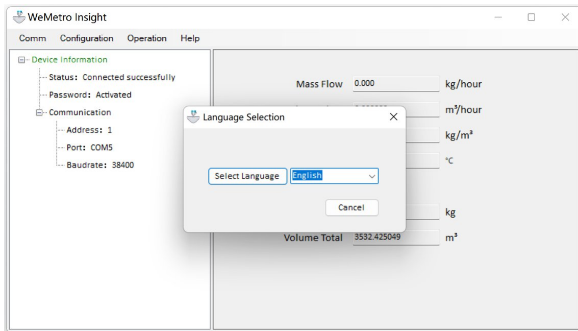
Рисунок 45 - HMI (интерфейс) меню «Language»
