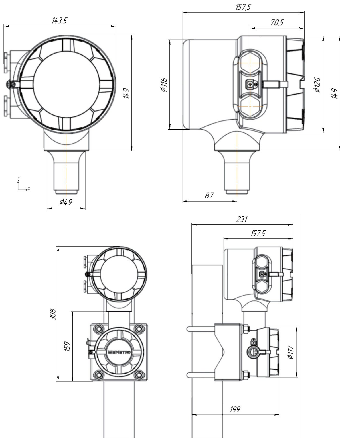
Рисунок 5 – Габаритные размеры преобразователей сигналов WMC-40 разнесённого и интегрального исполнений
