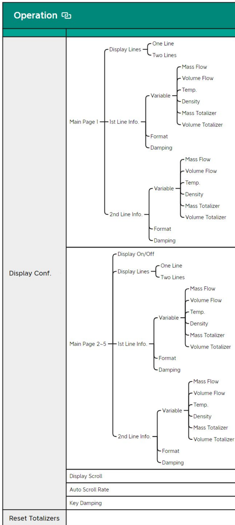
Рисунок 18 - Общая структура меню «Operation»
