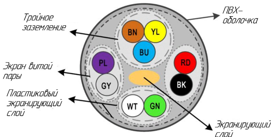
Рисунок 9 – Сечение соединительного межблочного кабеля
