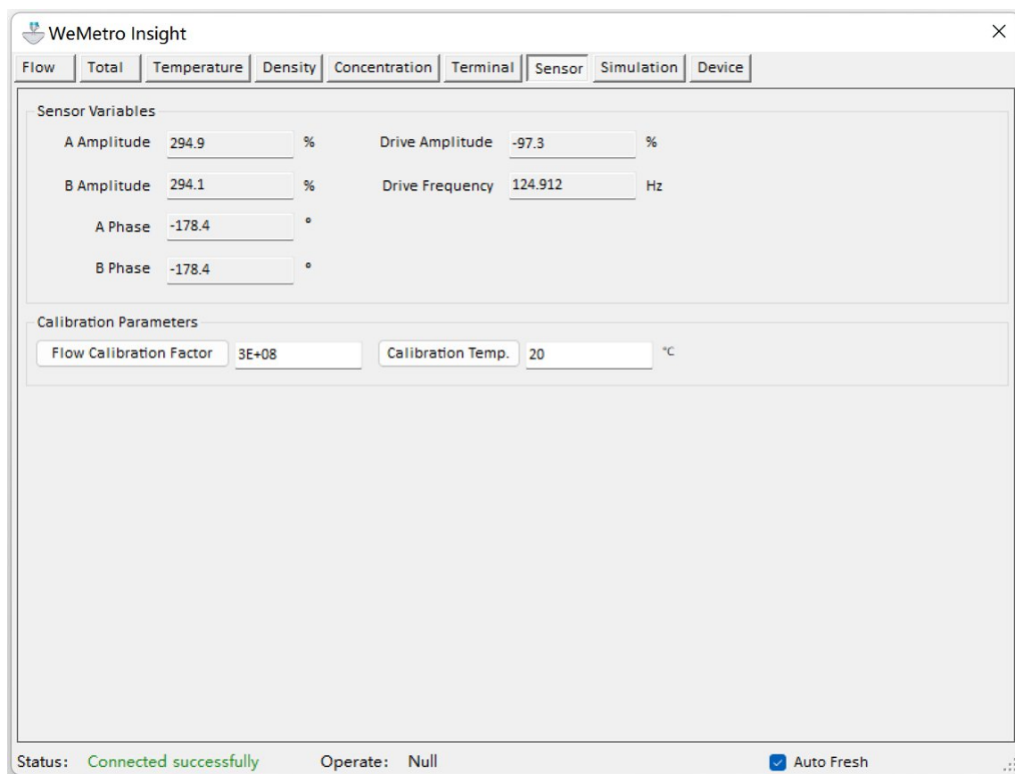
Рисунок 38 - НМИ (интерфейс) меню «Sensor»
