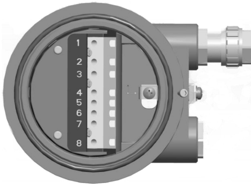
Рисунок 10 – Клеммная коробка без крышки
