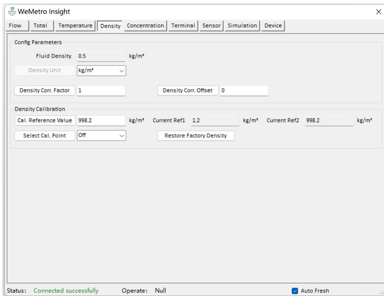
Рисунок 35 - НМИ (интерфейс) меню «Density»
