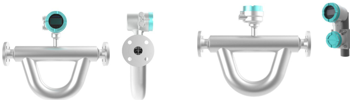
интегральное исполнение расходомера с преобразователем сигналов WMC-40I
