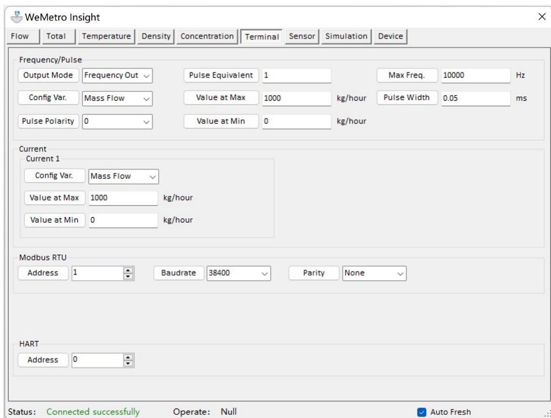
Рисунок 37 - HMI (интерфейс) меню «Terminal»
