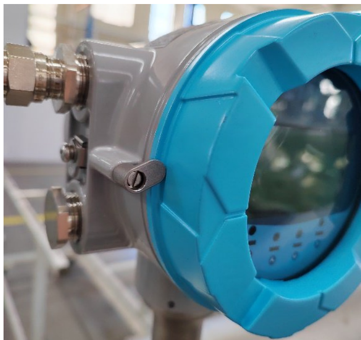
Рисунок 2 – Фиксатор крышки преобразователя сигналов WMC-40
