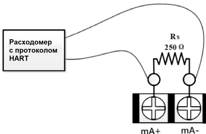
Рисунок 46 - Соединение HART с активной токовой петлей
