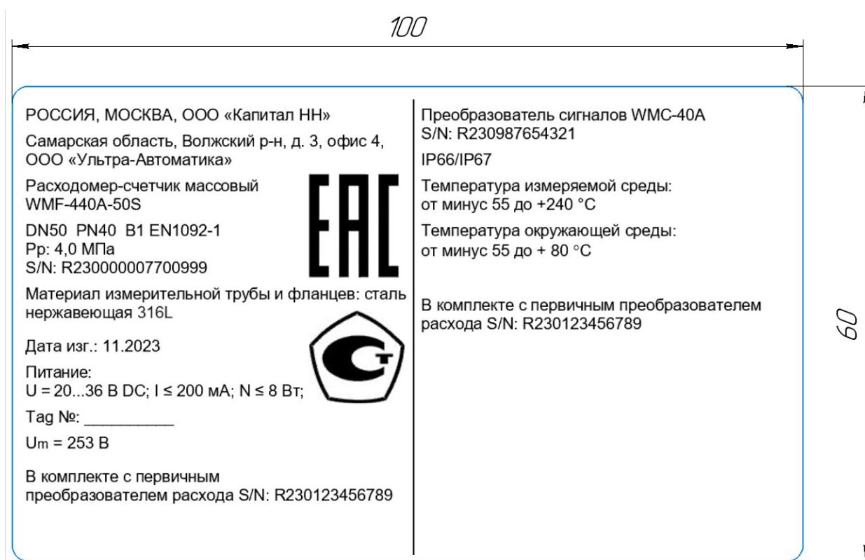
Рисунок 6 – Пример паспортной таблички на корпусе преобразователя сигналов WMC-40
