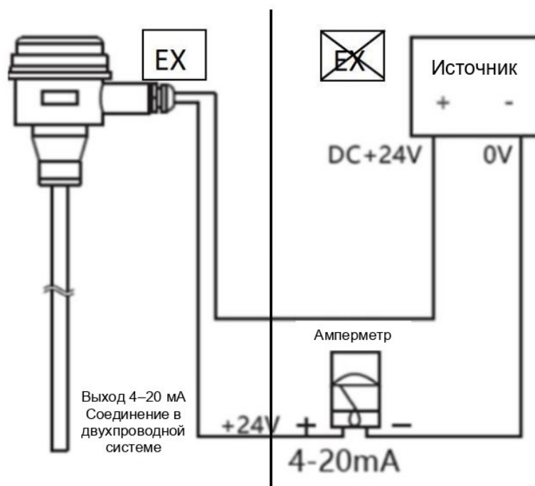
Рисунок 2 – Установка уровнемера
